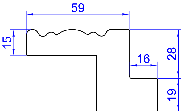
Z DECO (4008)
